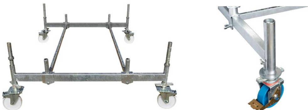
Fig. 46. Montarea bazei schelei și fixarea roților
